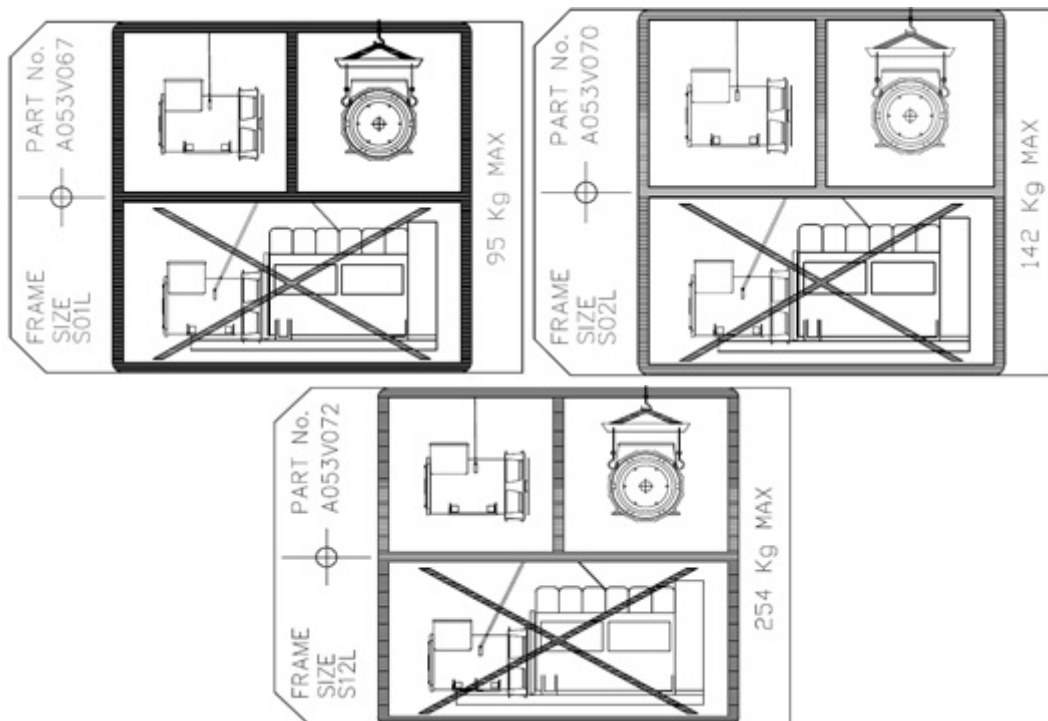
RYСУNEK 17. ETYKIETY PRZEDSTAWIAJĄCE SPOSÓB PODNOSZENIA ALTERNATORA
