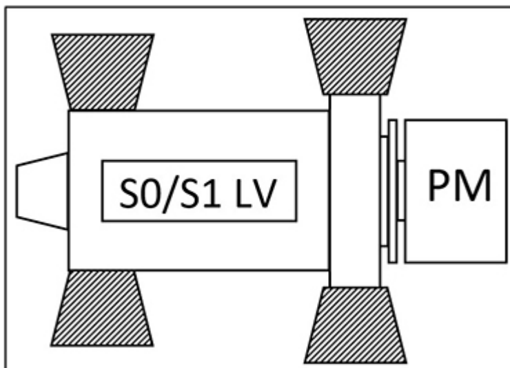
RYSUNEK 5. STREFY ZAGROŻENIA WOKÓŁ ALTERNATORA S0 I S1
