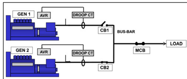
FIGURA 12. ALTERNATORI IN PARALLELO O A SINCRONIZZAZIONE
