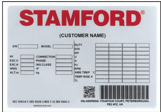
FIGURA 3. TARGA DATI OPERATIVI INTERNAZIONALE DELL'ALTERNATORE C.A. STAMFORD
