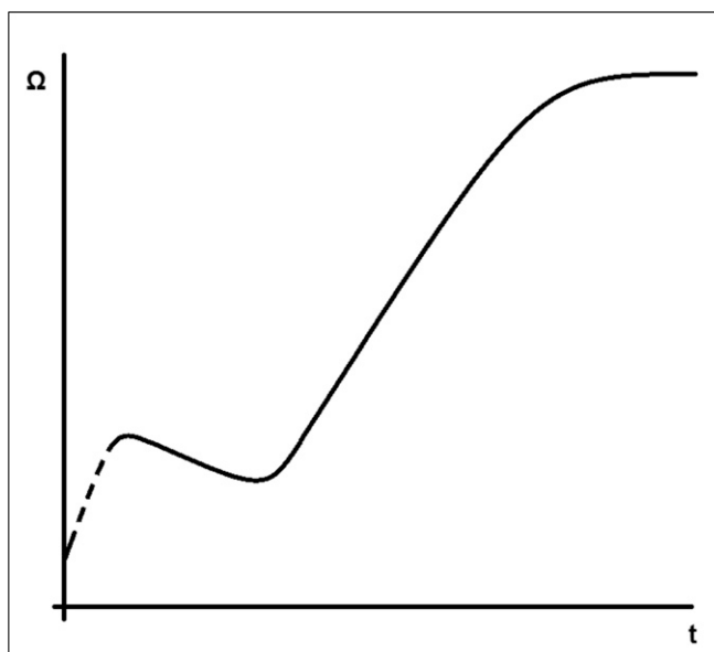
FIGURA 14. GRAFICO RESISTENZA DI ISOLAMENTO
