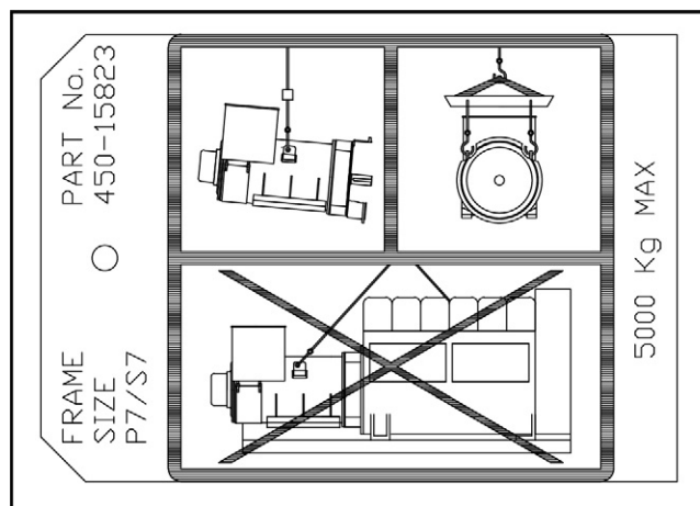
FIGURA 7. ETICHETTA CON CONFIGURAZIONE DI SOLLEVAMENTO
