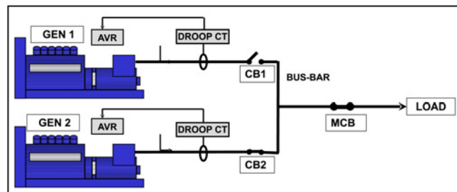
FIGURE 12. ALTERNATEURS PARALLÈLES OU DE SYNCHRONISATION
