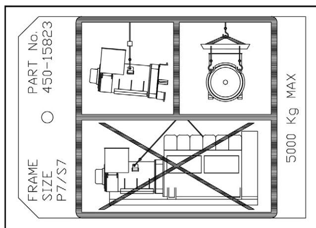
FIGURE 7. ÉTIQUETTE DE LEVAGE
