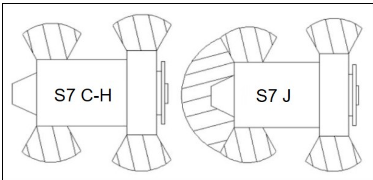
FIGURE 1. ZONES ÉCLOSES
