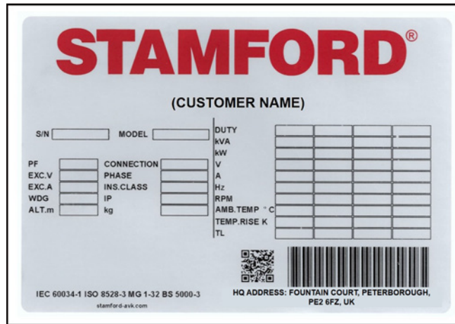
FIGURE 3. PLAQUE SIGNALÉTIQUE DES ALTERNATEURS C.A. GLOBAL STAMFORD
