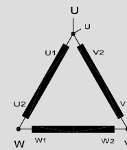
Delta 3Ph 4W Output Terminals (U.V.W.)
