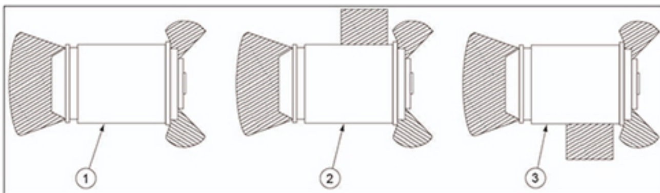
FIGURE 5. ZONES DE DANGER DE L'ALTERNATEUR S9
