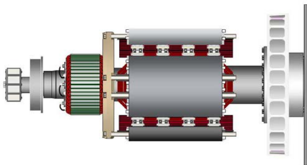
FIGURE 20. ROTOR DE L'ALTERNATEUR À PALIER SIMPLE MONTRANT LES DISQUES D'ACCOUPLMENT BOULONNÉS À LA COURSE D'ACCOUPLMENT À L'EXTRÉMITÉ MOTRICE (À DROITE)
