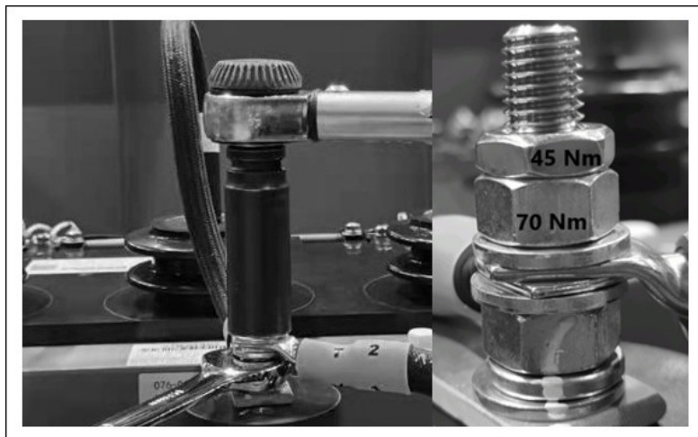
FIGURE 25. SERRE-CÂBLES CORRECTS (CÂBLES MULTIPLES)
