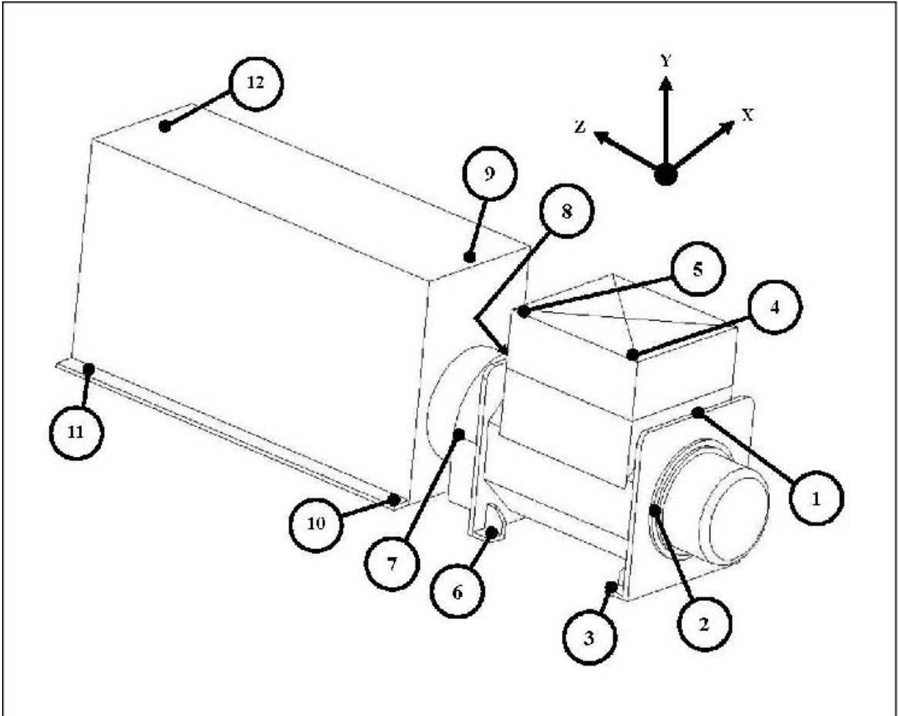
FIGURE 17. POSITIONS DE MESURAGE DES VIBRATIONS
