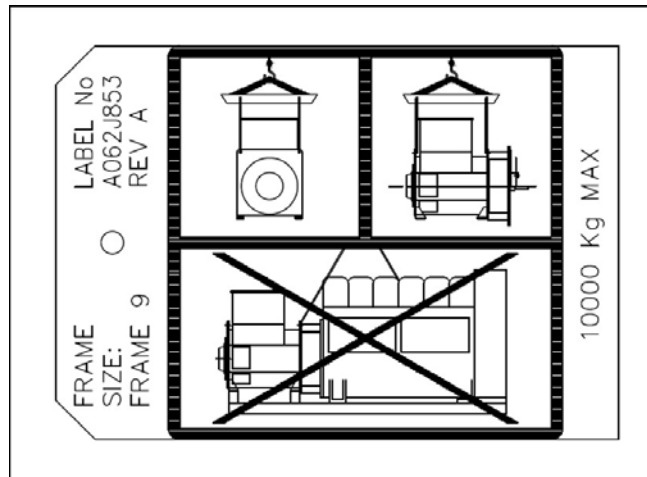
FIGURE 18. ÉTIQUETTE DE LEVAGE
