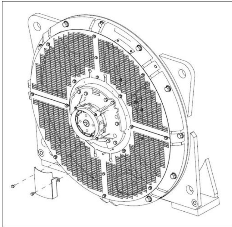
FIGURE 27. PURGEUR DE GRAISSE S9
