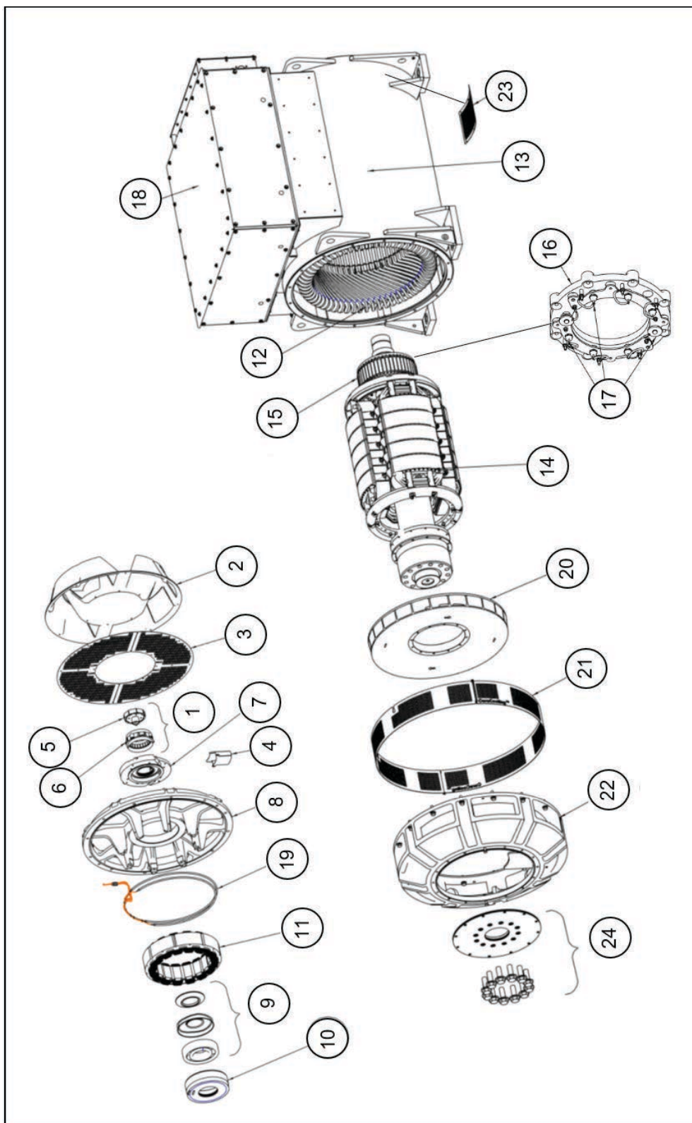
FIGURE 30. ALTERNATEURS S9 À PALIER SIMPLE
